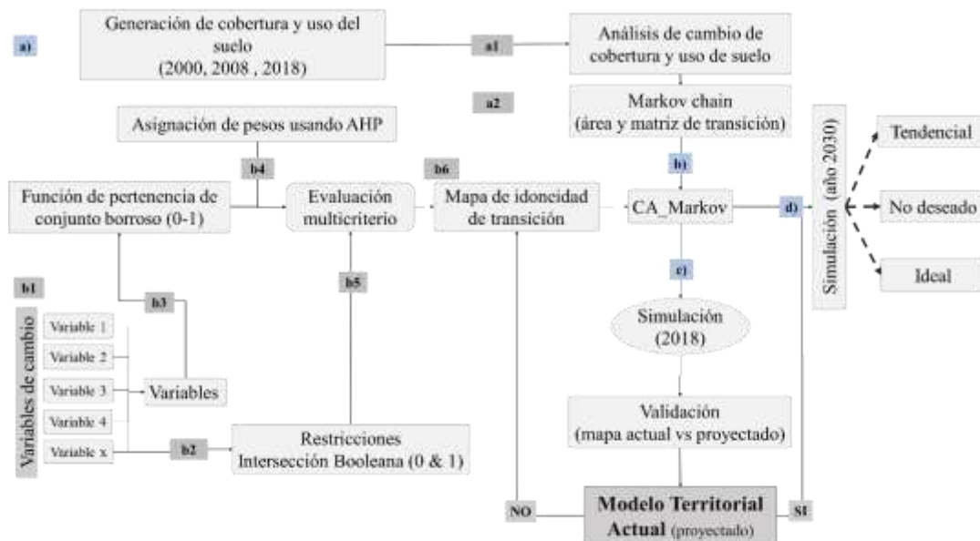
Figura 1. Diagrama esquemático para simular el cambio uso de suelo 4 a futuro usando el modelo CA_Markov.
