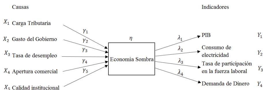
GRÁFICO 1: Diagrama de ruta del modelo MIMIC Elaboración propia
