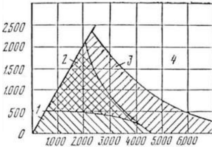
Figura 27: Elección del esquema o tipo de intersección. Fuente: (Ministerio de Transporte y Obras Públicas, 2003: 4A).
