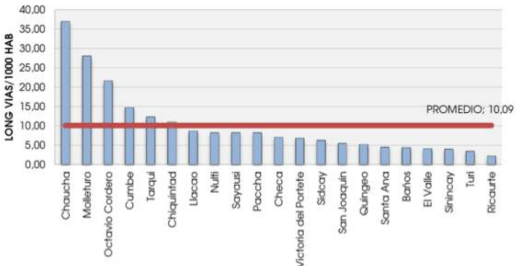
Figura 22: Promedio de longitud vial por parroquia por cada 1000 habitantes, cantón Cuenca.
