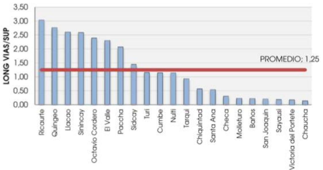
Figura 21: Densidad vial por parroquia, cantón Cuenca. Fuente: (Flores, 2013: 92).
