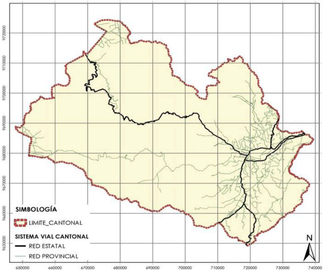
Figura 14: Vías cantonales, cantón Cuenca.
