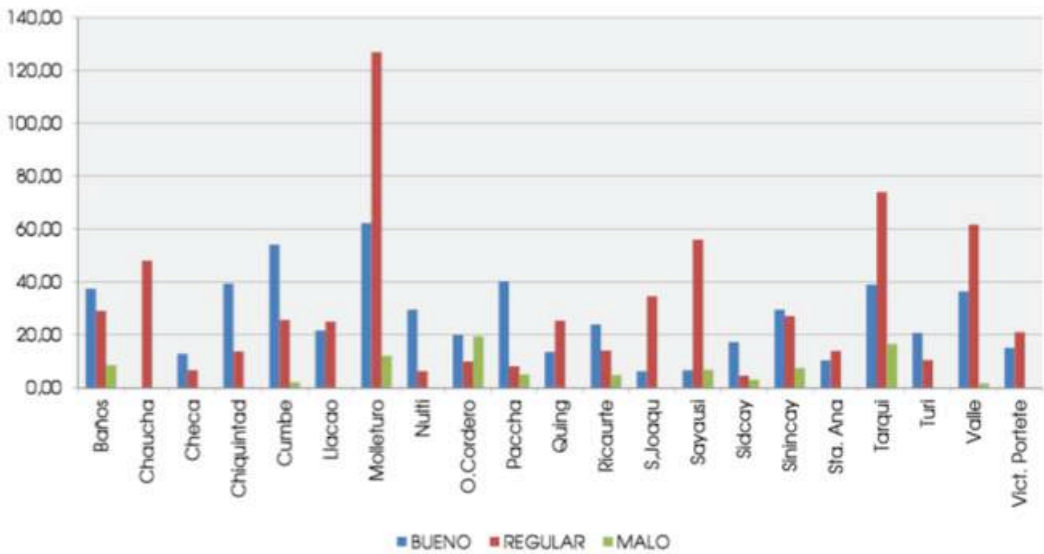
Figura 18: Estado de las vías por parroquia, cantón Cuenca. Fuente: (Flores, 2013: 93).
