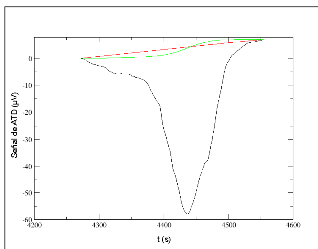
Figura 3. Pico de calentamiento del \text{AgIn}_5\text{S}_8 a 15\text{ }^\circ\text{C}/\text{min} . El eje vertical es la señal de ATD en \mu\text{V} , el eje horizontal es el tiempo en segundos. La línea verde representa la línea base corregida.
