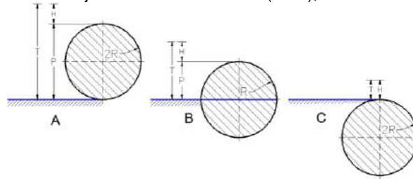
Fig. 1.- Vertedero de perfil circular en las tres posiciones ensayadas.
