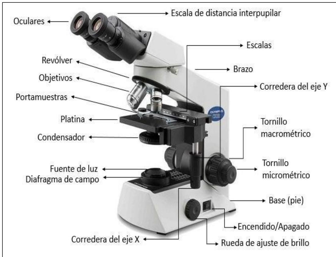
Ilustración 2. Partes del microscopio óptico compuesto. Tomado y modificado de (20).
