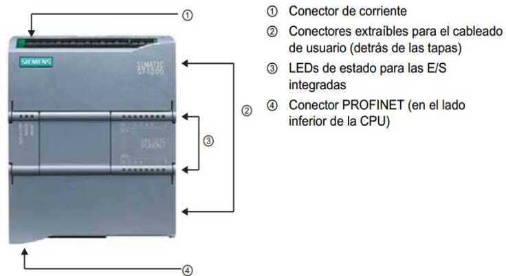
FIG.15b PLC Siemens S7-1200 21
