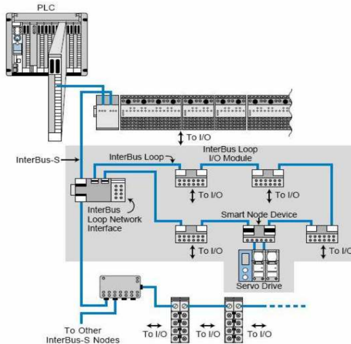
FIG.5 Redes: InterBus Loop e InterBus-S interconectadas 5
