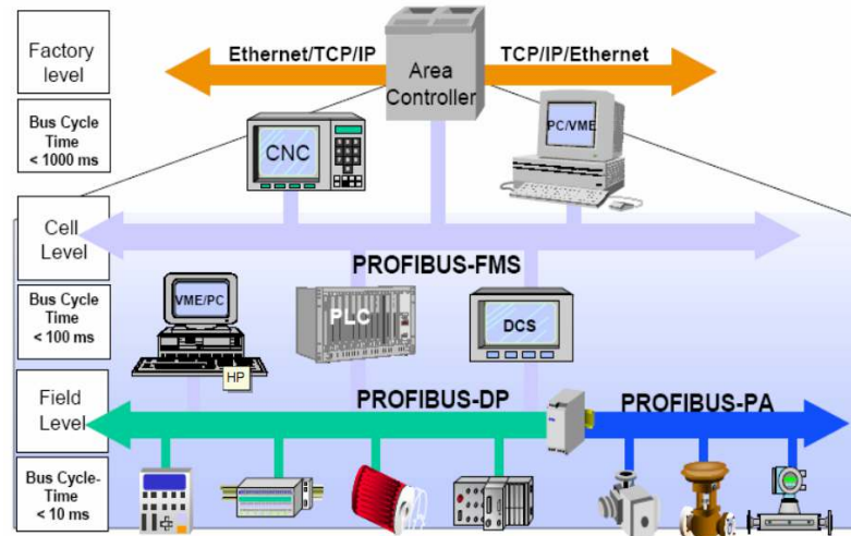
FIG.8 Red de Procesos Profibus 8
