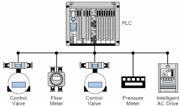
FIG.7 Configuración de una Red de Procesos 7
