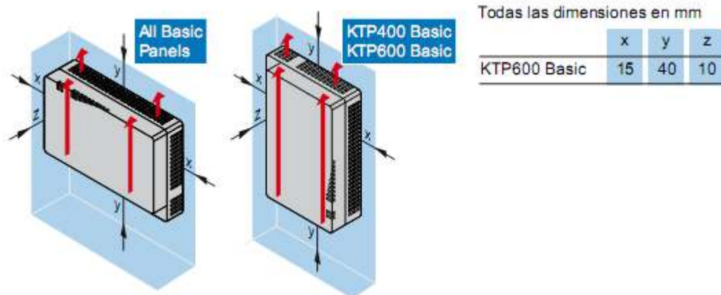
FIG.111 Distancias de separación alrededor del panel de operador 40
