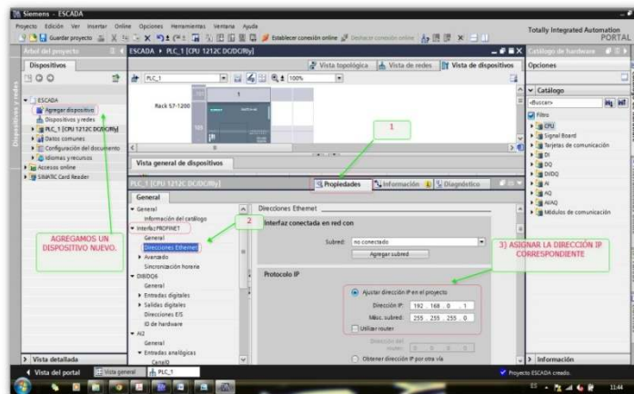
FIG.40 Configuración de la IP del PLC_1
