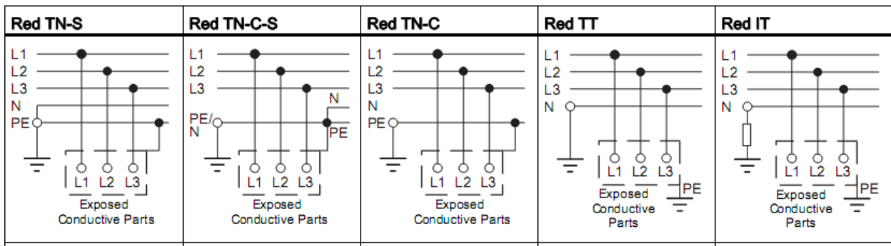
FIG.107 Sistemas de distribución de corriente 36
