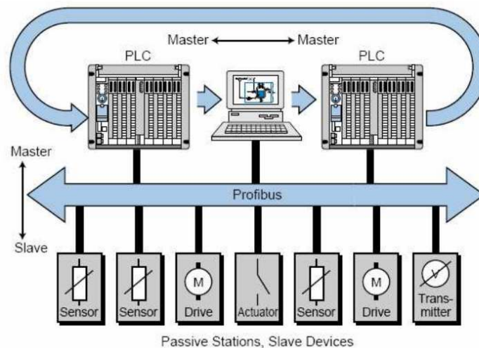
FIG.11 Comunicaciones maestro-esclavo y maestro-maestro en una red Profibus 13
