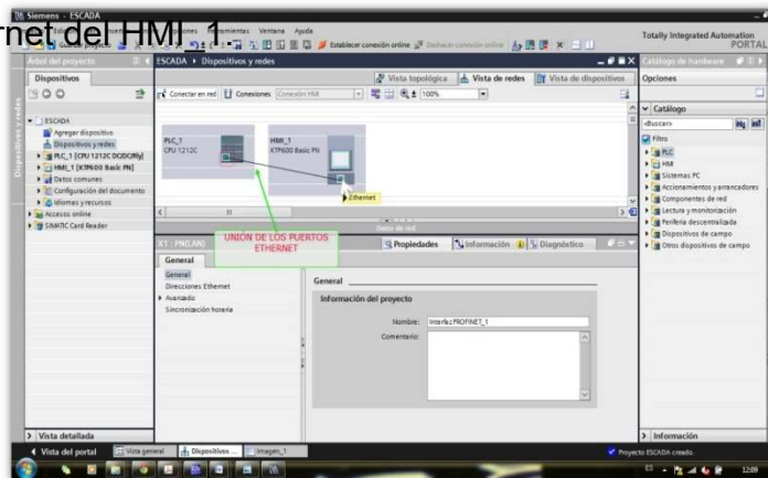
FIG.44 Enlace de comunicación Ethernet entre PLC_1 y HMI_1
