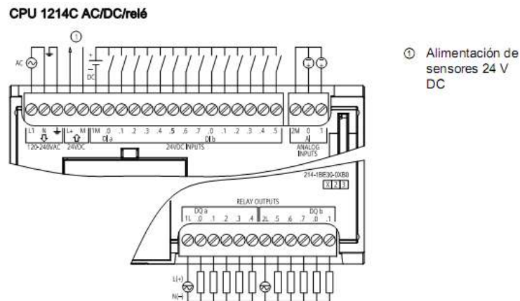
FIG.103 Diagramas de cableado para la CPU S7-1200 32
