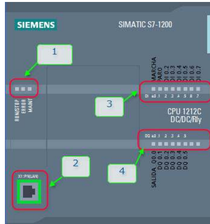
FIG.31 Vista del PLC S7-1200 con sus partes empleadas para la programación de la red; 1) Leds indicadores de estado (RUN/STOP/ERROR); 2) Puerto Ethernet; 3) Leds de estado de entradas digitales (I0.0,... I0.7); 4) Leds de estado de salidas digitales (Q0.0,... Q0.7)
