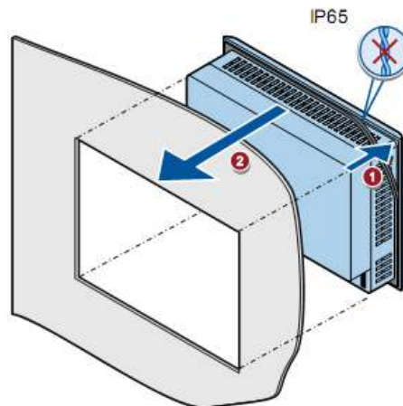
FIG.113 Montaje del HMI KTP600 Basic Color PN 42
