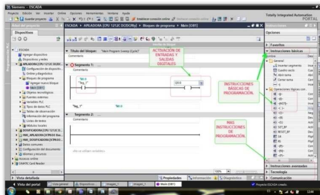
FIG.49 Programación de la lógica del PLC_1 (S7-1200 AC/DC)
