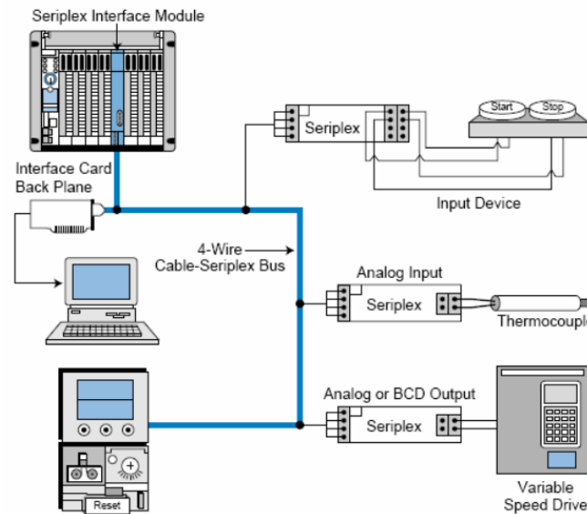
FIG.6 Red Seriplex con Controlador de Tráfico 6
