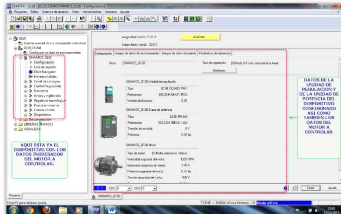
FIG.90 Ingreso de los Datos y Características del Motor
