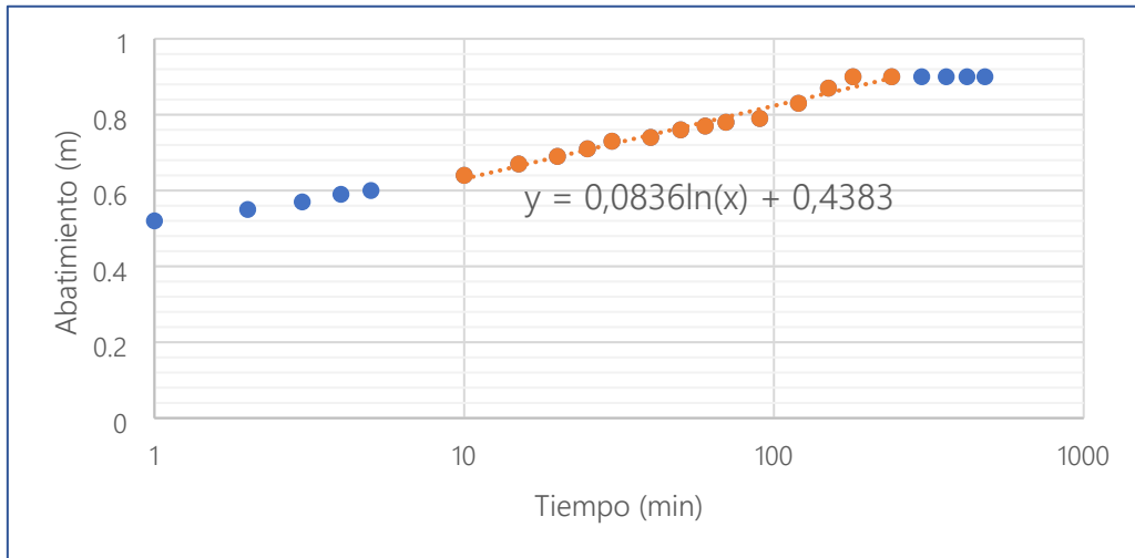
Figura 4-12. Nivel dinámico vs tiempo - pozo de observación RM-02
