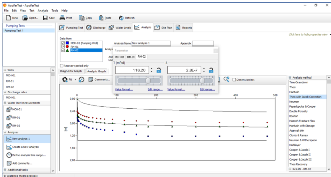
Figura 4-21. Transmisividad y coeficiente de almacenamiento RM-01. AquiferTest2016.1
