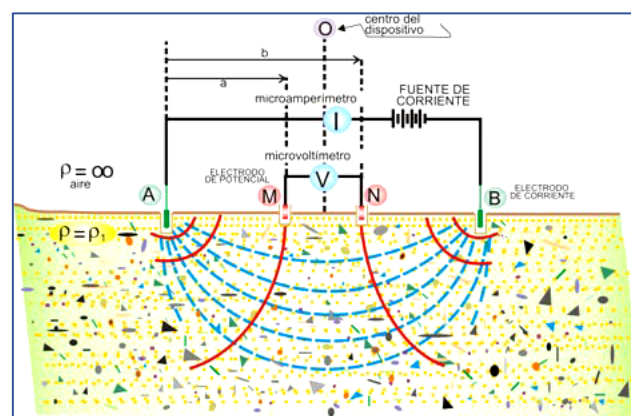
Figura 2-3. Medida de la resistividad aparente, en dos estratos de diferente resistividad
