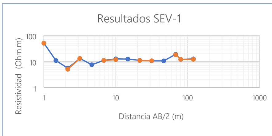
Figura 4-1. Resultados Sondeo Eléctrico Vertical 1
