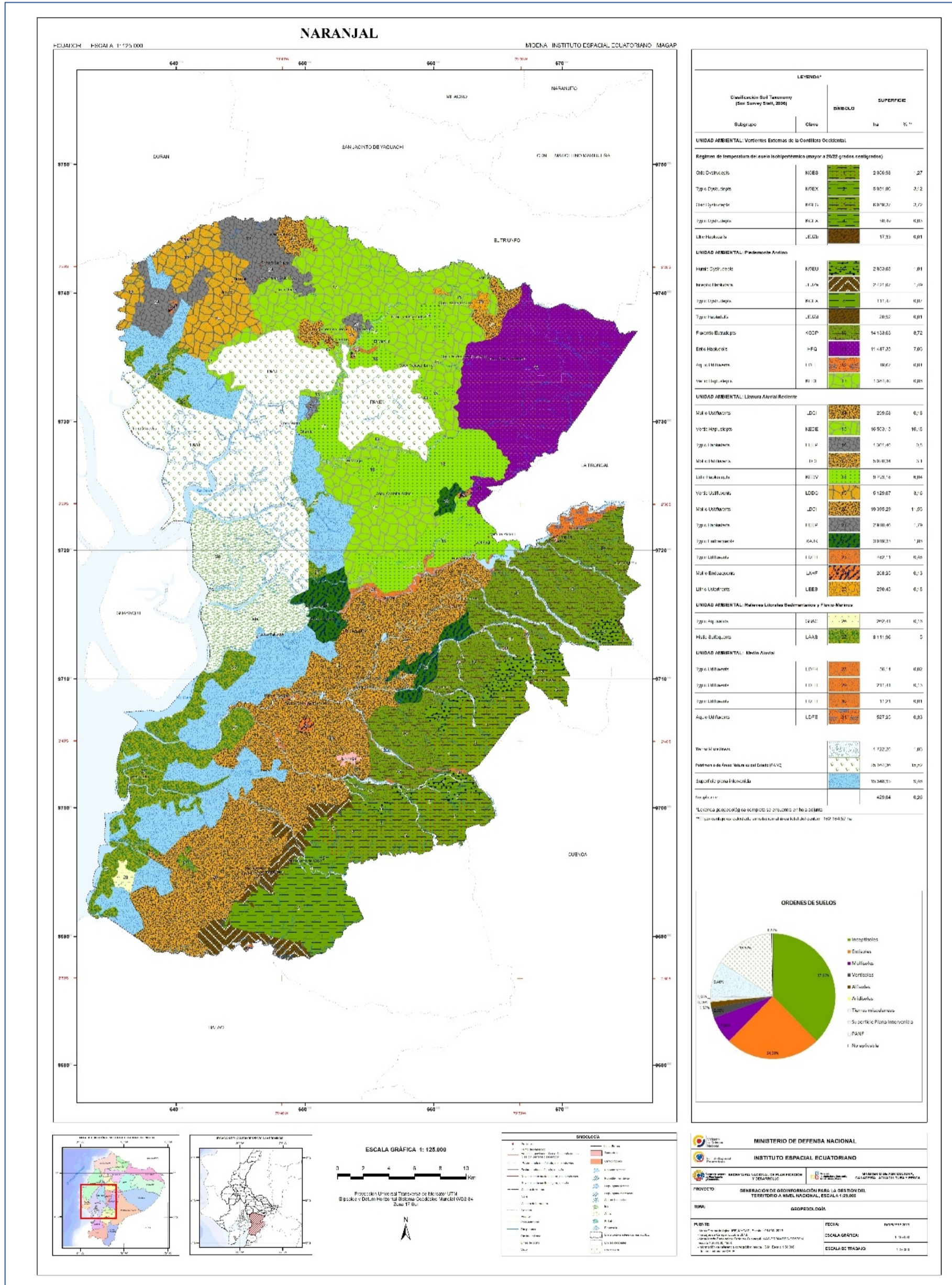
Figura 3-8. Mapa Geopedológico del cantón Naranjal
