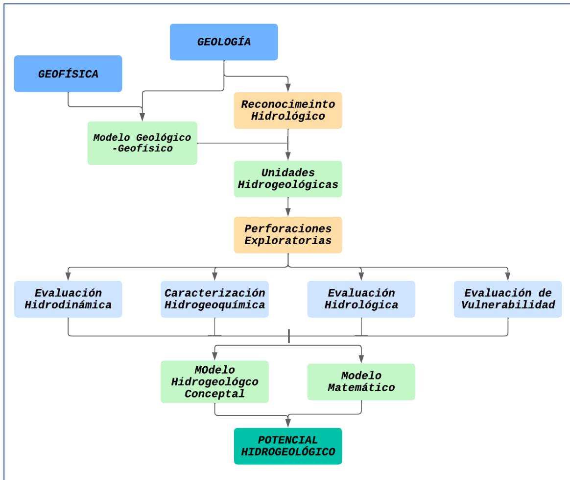
Figura 2-1. Flujo diagrama conceptual para la exploración hidrogeológica.
