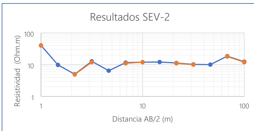
Figura 4-2. Resultados Sondeo Eléctrico Vertical 2
