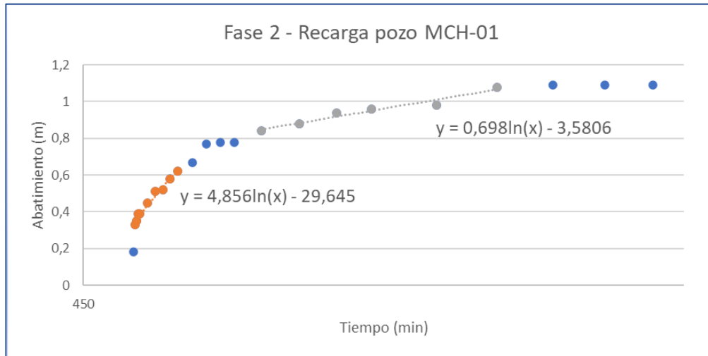
Figura 4-8. Recuperación vs tiempo - pozo exploratorio MCH-01
