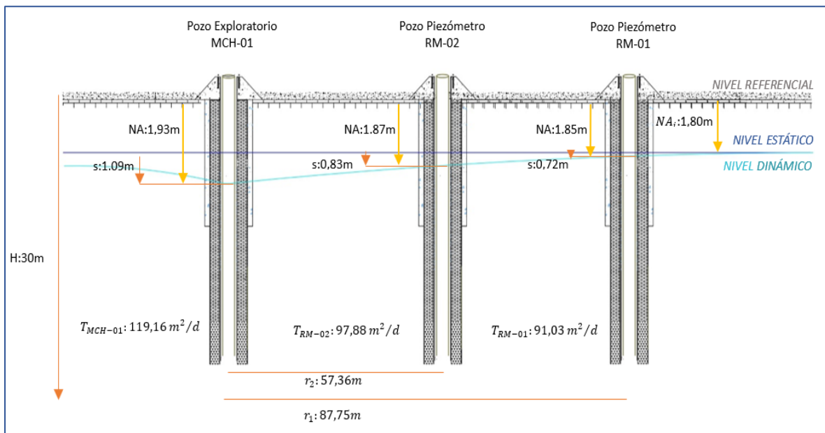
Figura 4-25. Esquema de los pozos en condiciones de recarga
