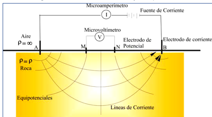
Figura 2-2. Circuito de emisión y recepción
