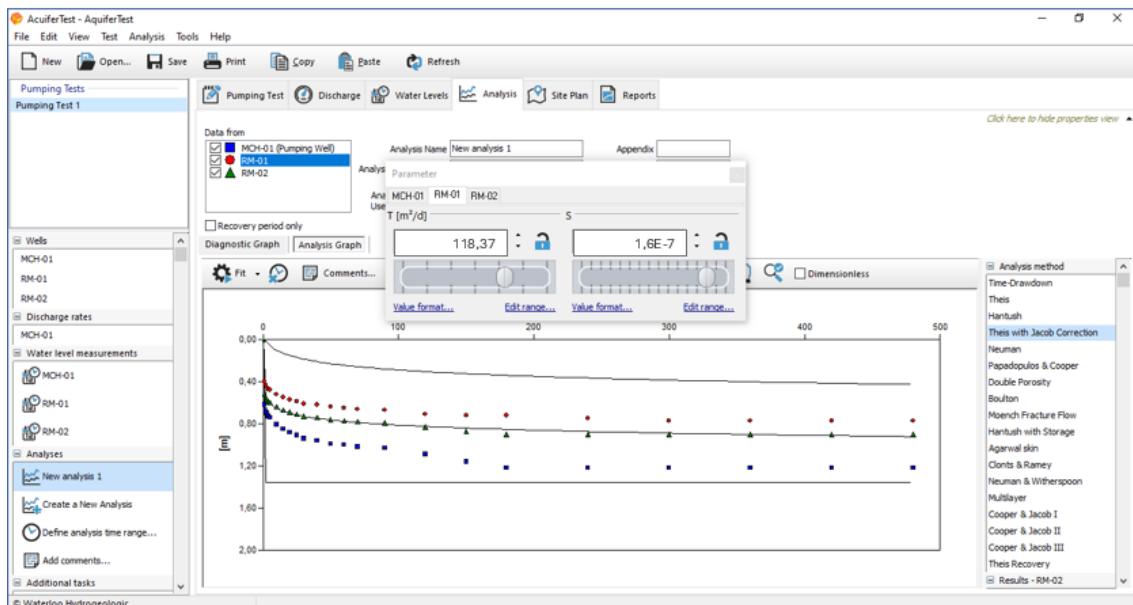
Figura 4-22. Transmisividad y coeficiente de almacenamiento RM-02. AquiferTest2016.1
