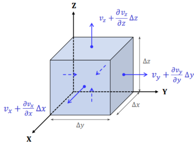
Figura 2-30. Elemento diferencial de un medio poroso. Condiciones de continuidad de flujo
