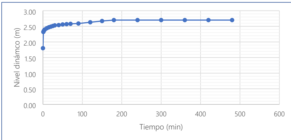
Figura 4-13. Abatimiento vs tiempo - pozo de observación RM-02
