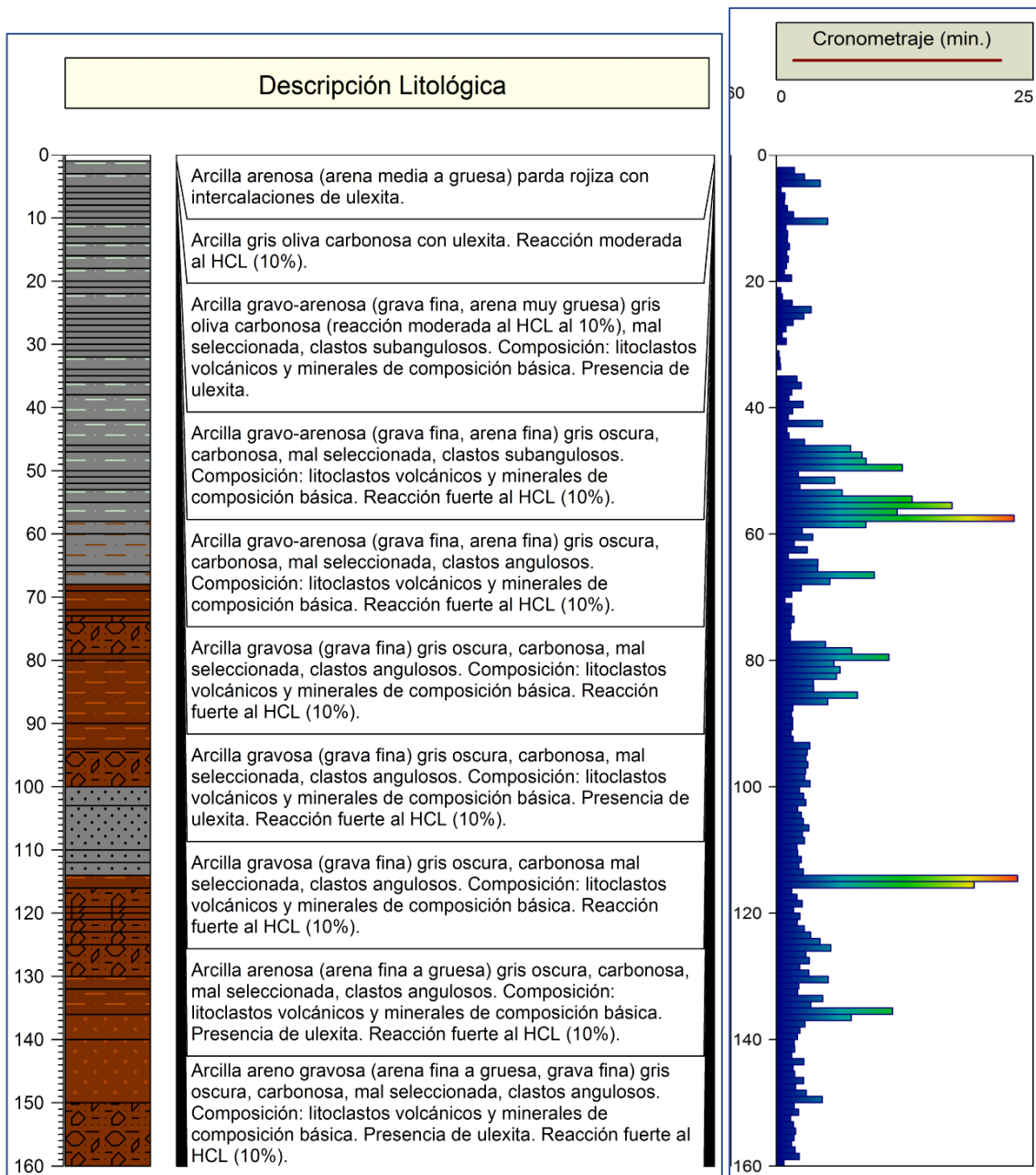
Figura 2-28. Perfil litológico y perfil de cronometraje en un pozo exploratorio
