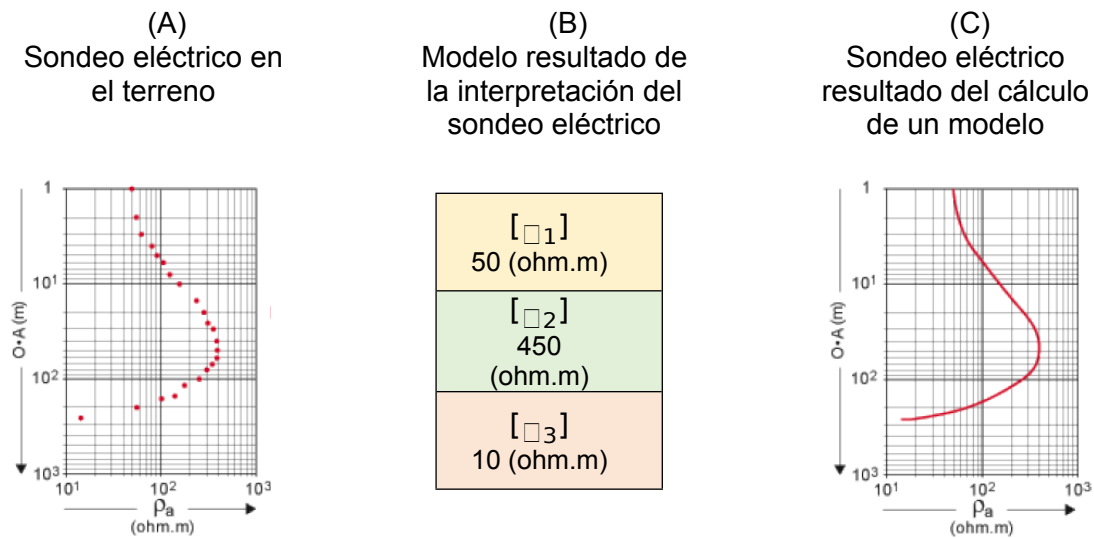
Figura 3-9. Proceso de inversión de datos de resistividad geoelectrica
