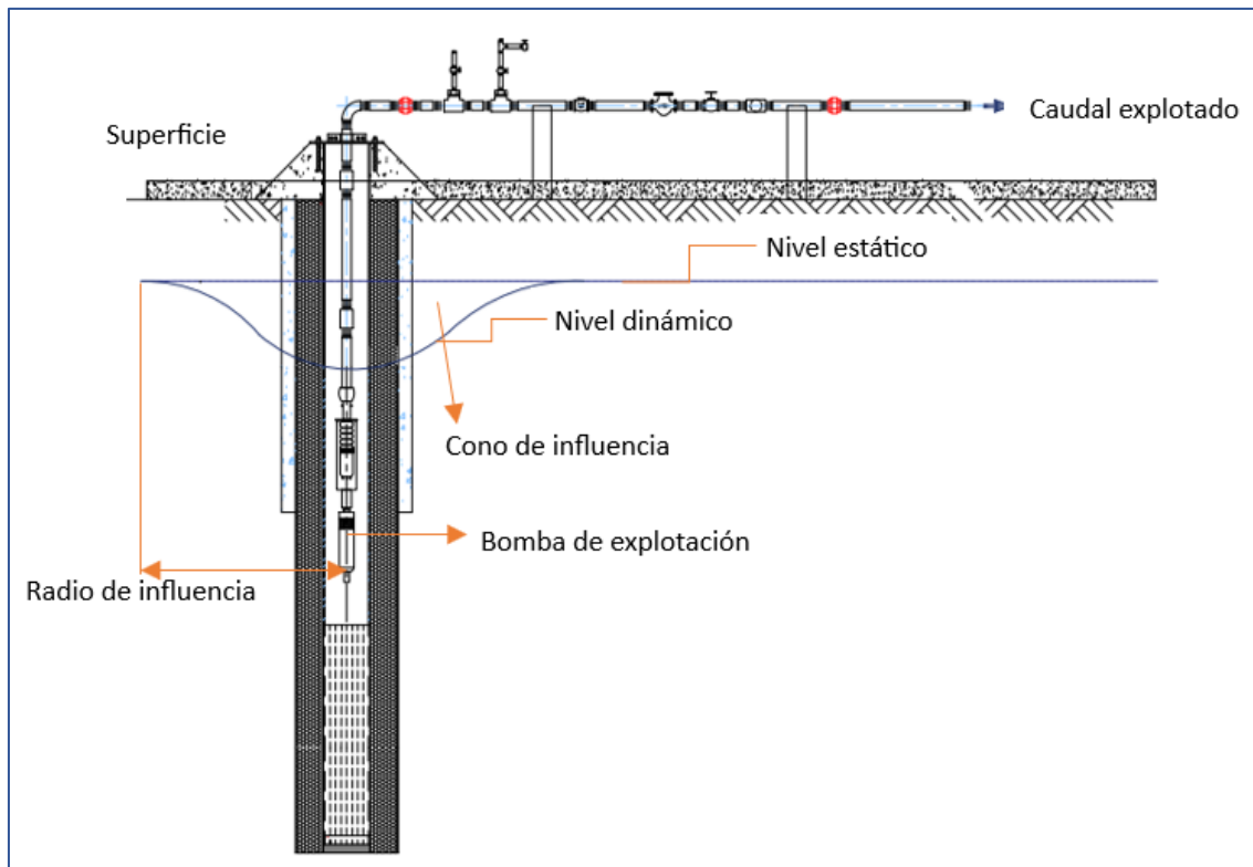
Figura 2-29. Cono de influencia al bombear un pozo de explotación
