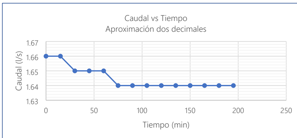
Figura 4-4. Tendencia del caudal en el tiempo (3horas con 15minutos)
