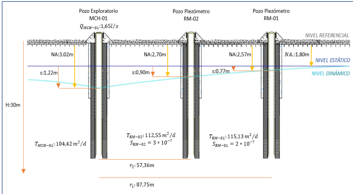
Figura 4-24. Esquema de los pozos en condiciones de bombeo
