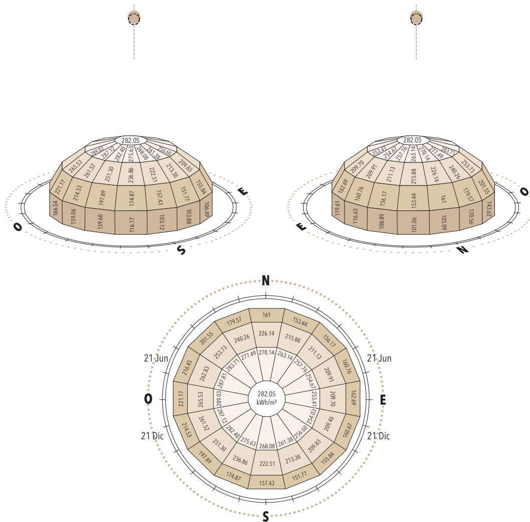
Figura 85. Producción eléctrica fotovoltaica esperada por m 2 en Manta, centro urbano (kWh/m 2 al año)
