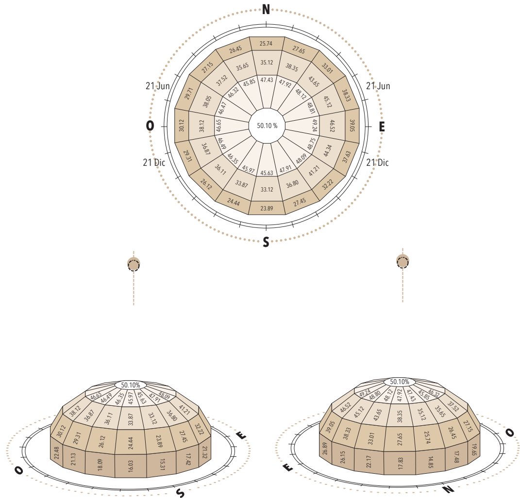
Figura 89. Fracción solar en % esperada por sistema solar térmico residencial con 2 m² en Quito (%)
