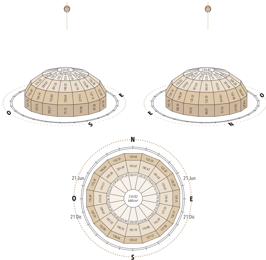
Figura 87. Producción eléctrica fotovoltaica esperada por \text{m}^2 en Machala, centro urbano ( \text{kWh/m}^2 al año)
