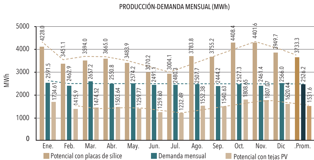
Figura 53. Generación eléctrica mensual frente a producción factible con placas fotovoltaicas de silicio y tejas fotovoltaicas [265]
