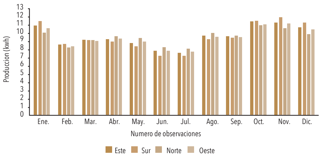
Figura 42. Producción mensual fotovoltaica de placa de 36 celdas, acorde a distintas orientaciones [222]
