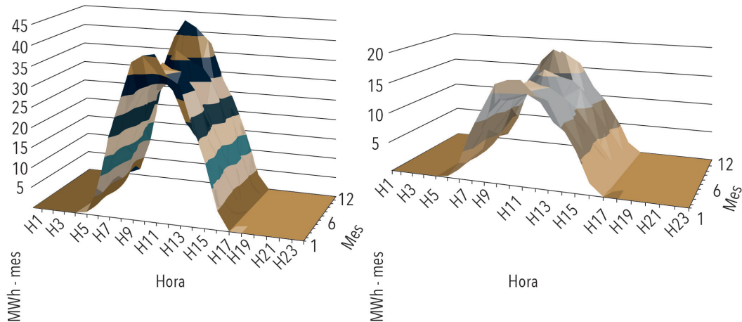
Figura 65. Producción de placas de silicio (izquierda) y tejas fotovoltaicas (derecha), con ocupación de captación en la totalidad de los faldones [267]
