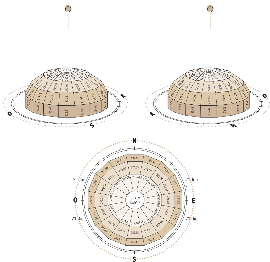
Figura 82. Producción eléctrica fotovoltaica esperada por \text{m}^2 en Riobamba, centro urbano ( \text{kWh/m}^2 al año)
