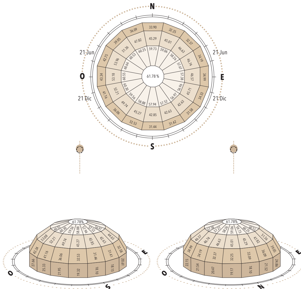
Figura 96. Fracción solar esperada por sistema solar térmico residencial con 2 \text{ m}^2 en Machala (%)
