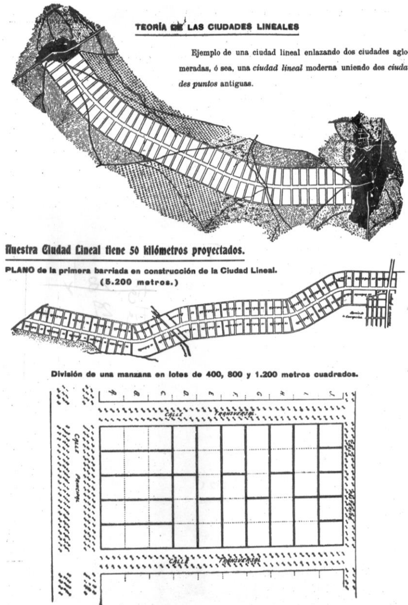
Figura 1: La C.L. uniendo dos ciudades "punto". Manzana y su división en parcelas o lotes. RCL 1898
