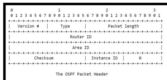
Figura 1. Formato del Encabezado de un paquete OSPFv3.
