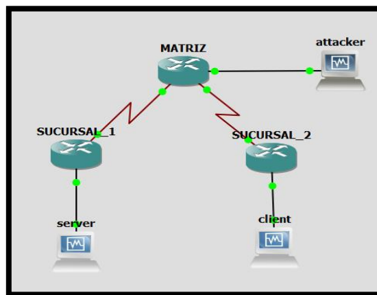
Figura 3: Esquema de red utilizado para ambos protocolos.
