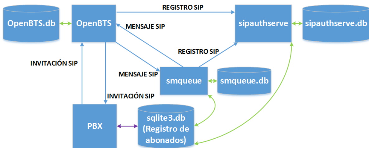
Figura 2. Diagrama del sistema OpenBTS.
