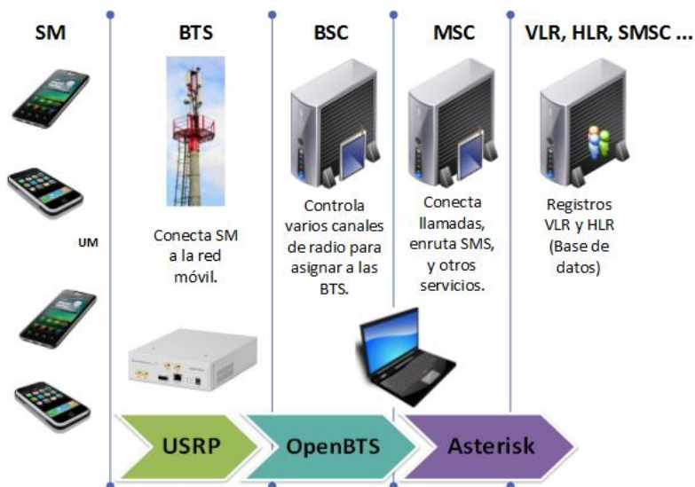
Figura 1. Arquitectura GSM comparado con OpenBTS.
