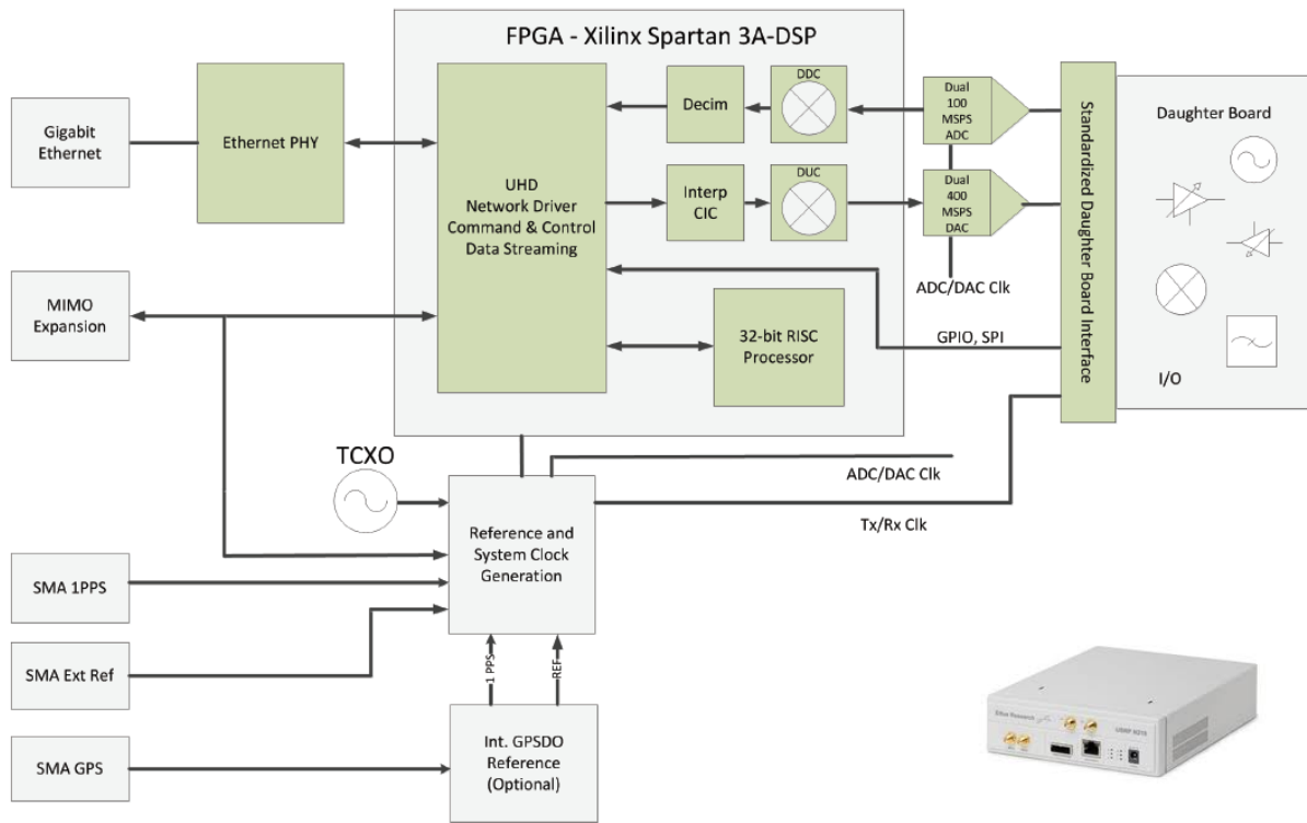
Figura 3. Arquitectura del USRP N210.
