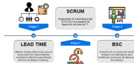
Fig 1: Metodología Propuesta.
