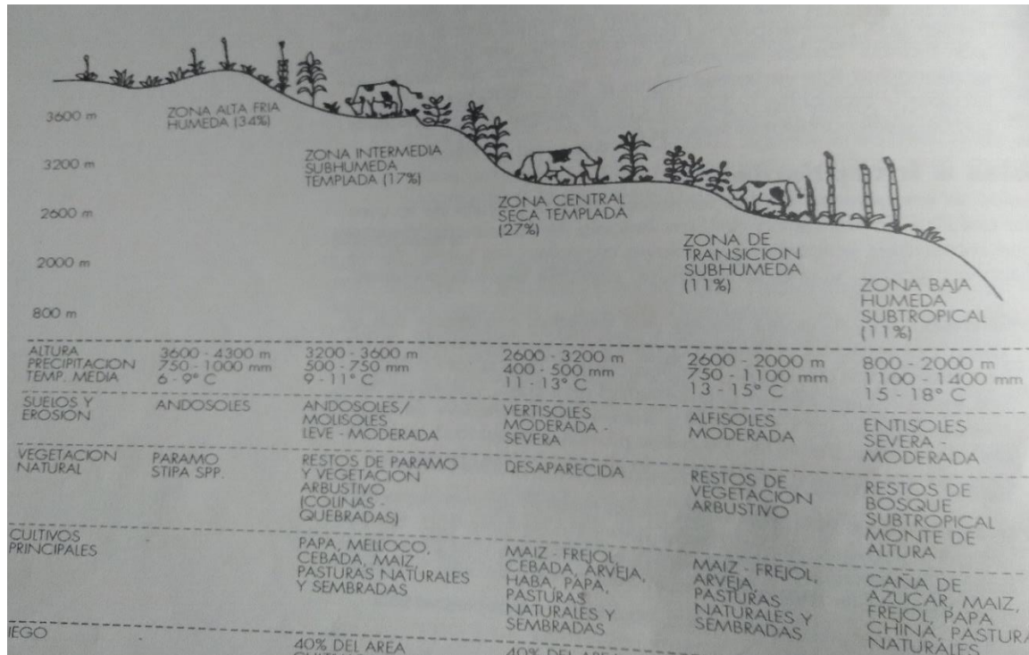
Grafico 4. Pisos ecológicos en la cuenca Alta del Rio Cañar
