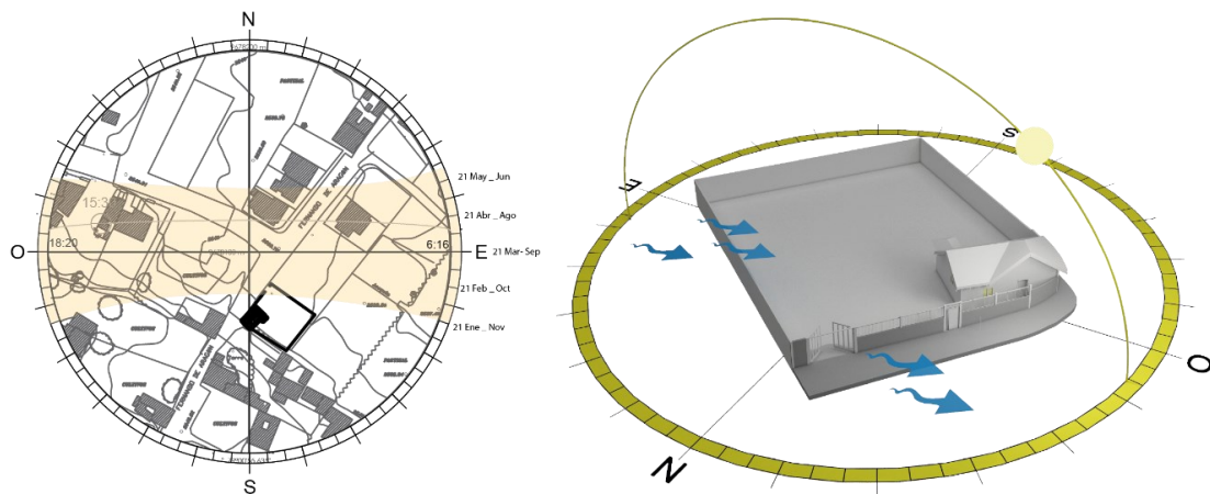
Figura 2. Recorrido del sol y corrientes de viento, Reinoso, E., 2019. Propuesta de diseño residencial mediante containers en la ciudad de Cuenca-Ecuador, para la familia Arévalo, Elaboración: Edwin Reinoso Y. (2019)
