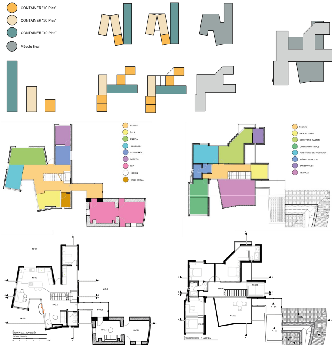
Figura 5. Distribución de espacios interiores, Reinoso. E, 2019, Propuesta de diseño residencial mediante containers en la ciudad de Cuenca-Ecuador, para la familia Arévalo, Elaboración: Edwin Reinoso (2019)
