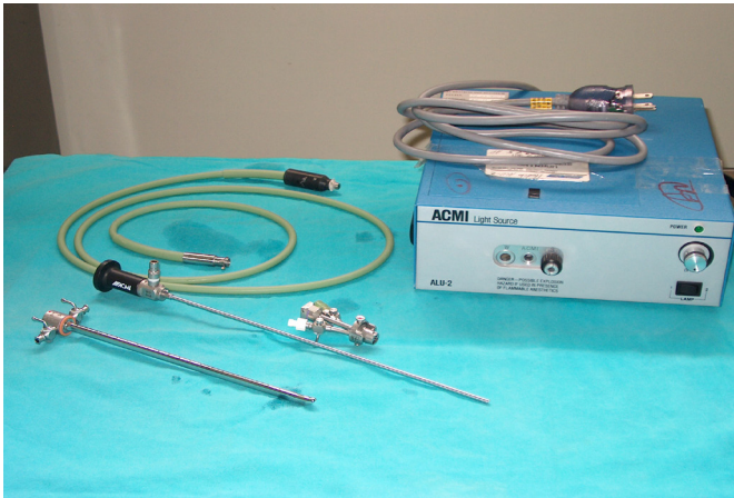
Fig.29. Fuente de Luz para cistoscopia
