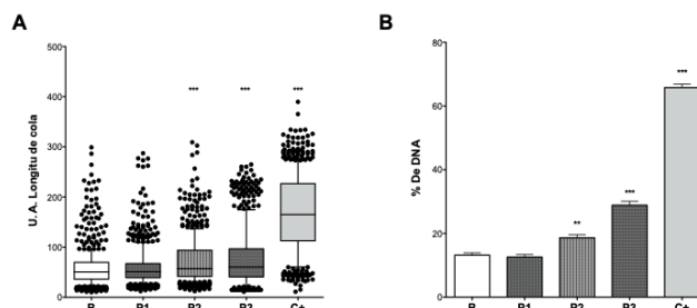
Figura 5: Efectos en el DNA en células CHO expuestas a los extractos acuosos (3,26 m 3 /mL). A. Longitud de la cola. B. % de DNA en la cola. Test Kruskal-Wallis y post test Dunns. Los datos representan 3 experimentos por duplicado. ** p < 0,001; *** p < 0,0001
