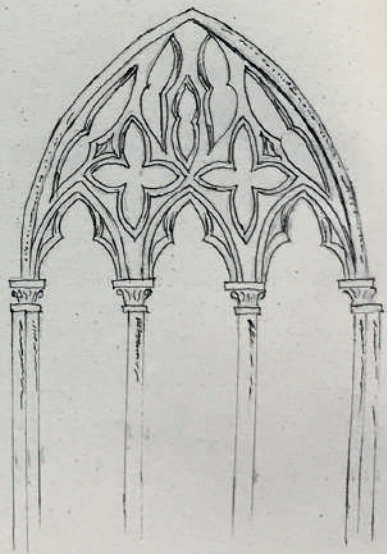
Tracería con elementos lobulados y nariz de tracería con dos mainel
