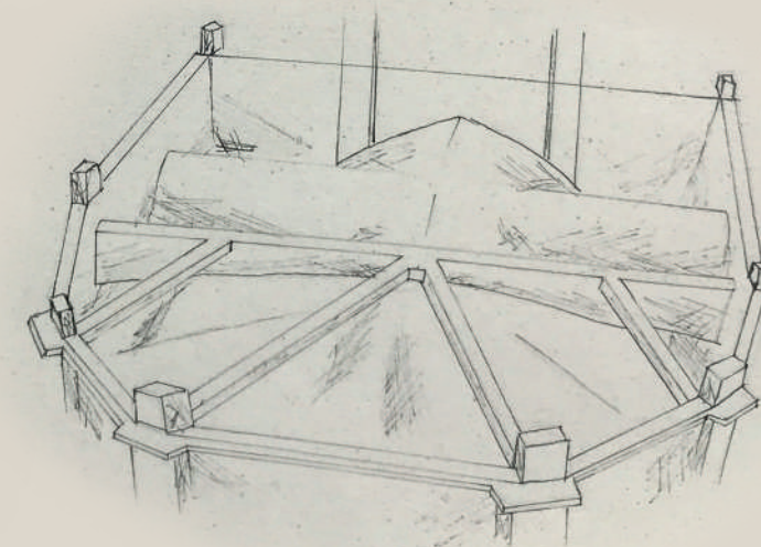
Bóveda de crucería sin cubierta de la cabecera
