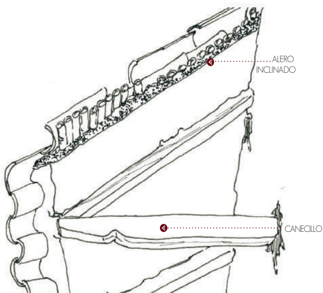
Imagen 37. Alero inclinado de barrio con canecillos
