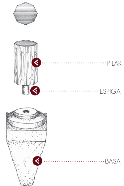
Imagen 10. Cimentación con piedra basa labrada.
