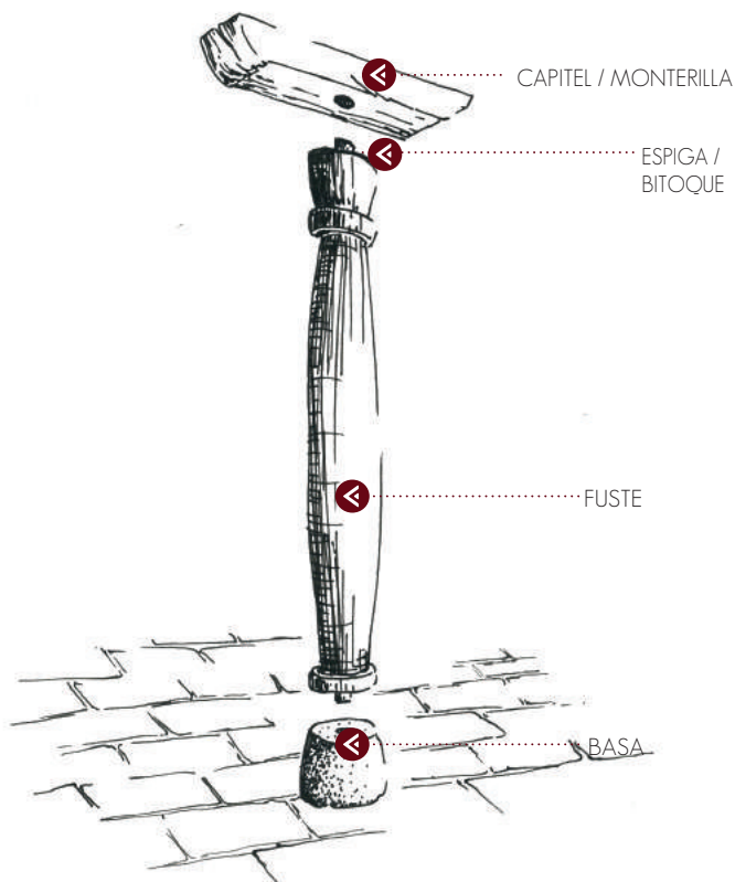
Imagen 16. Fuste de sección "panza".
