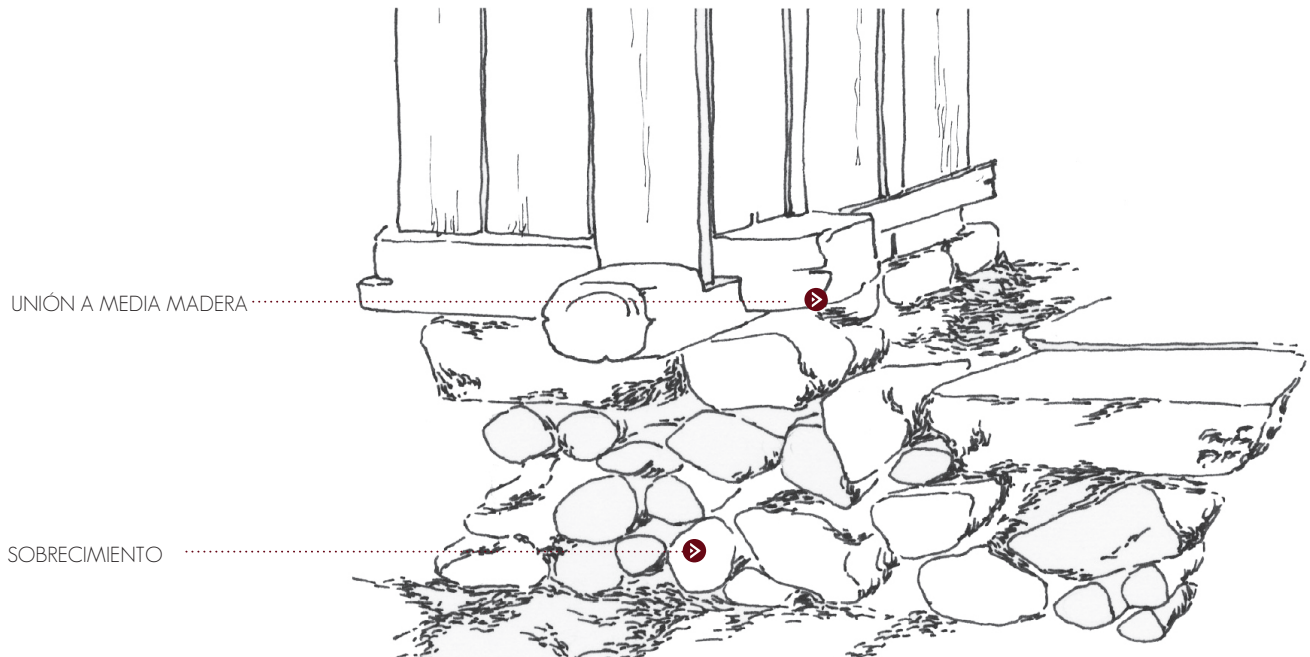
Imagen 11. Sobrecimiento.
