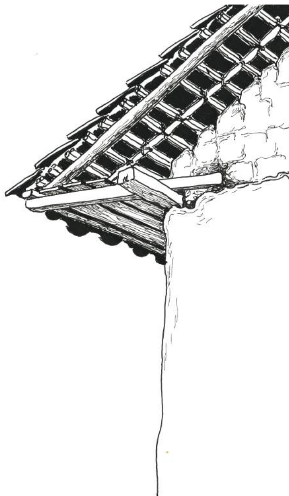
Imagen 41 . Alero sin canecillos a la vista.
