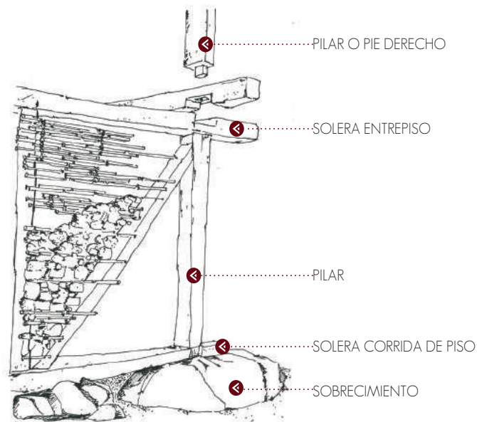
Imagen 12. Sistema de amarre de solera de entrepiso de madera.
