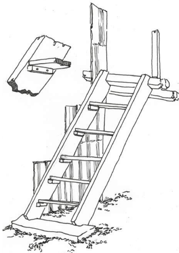
Imagen 68. Detalle de escaleras de madera.
