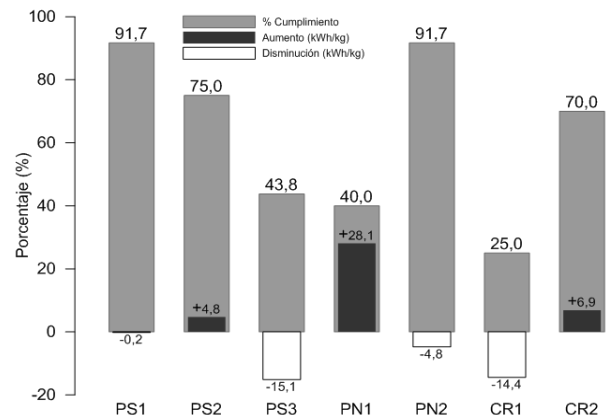
Figura 3. Relación % cumplimiento versus % reducción de consumo específico
